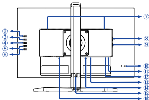
<Вид сзади>
