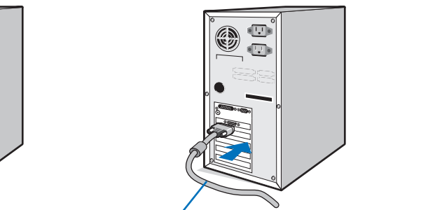
Сигнальный кабель с 15-контактным разъемом mini D-Sub Рисунок A.3
