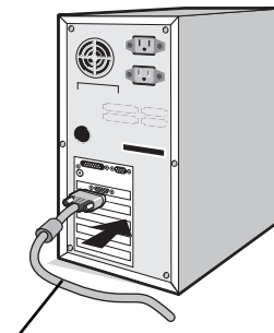
Кабель видеосигнала с 15-контактным разъемом mini D-SUB
