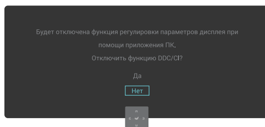
Рис. 40. Предупреждение DDC/CI
