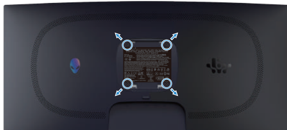
Рис. 27. Настенное крепление VESA
