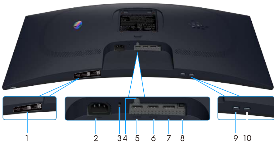
Рис. 3. Вид монитора снизу
