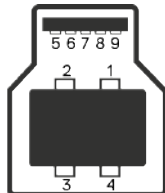
Рис. 6. Восходящий порт USB Type-B.
