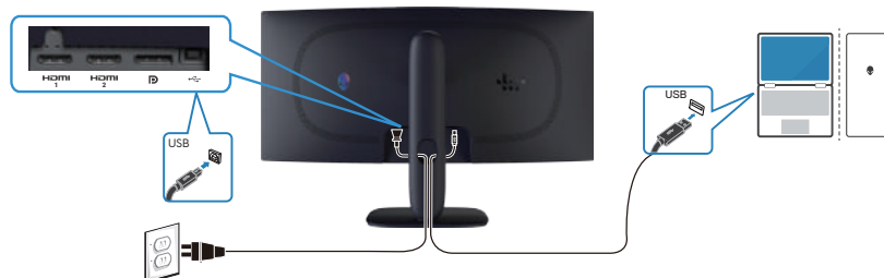
Рис. 24. Подключение кабеля USB Type-B (Type-B - Type-A)
