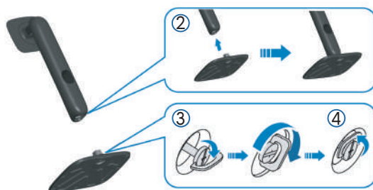
Рис. 13. Прикрепите подставку к основанию
